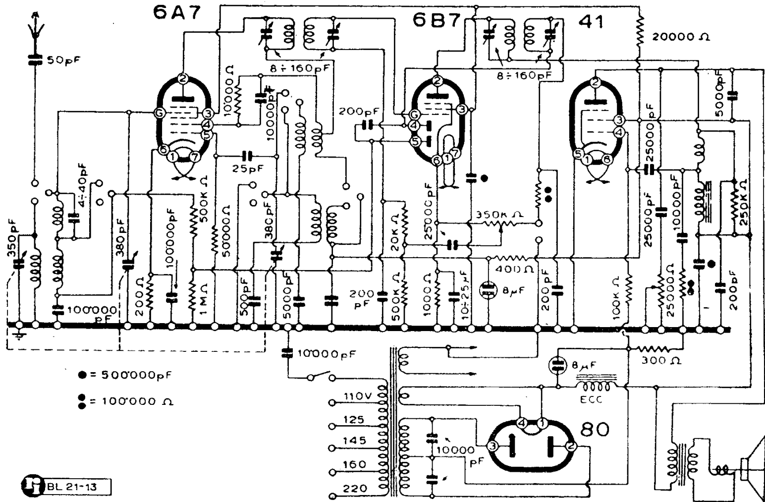
OFFICINE DI SAVIGLIANO - MOD. « 4 VALVOLE »
